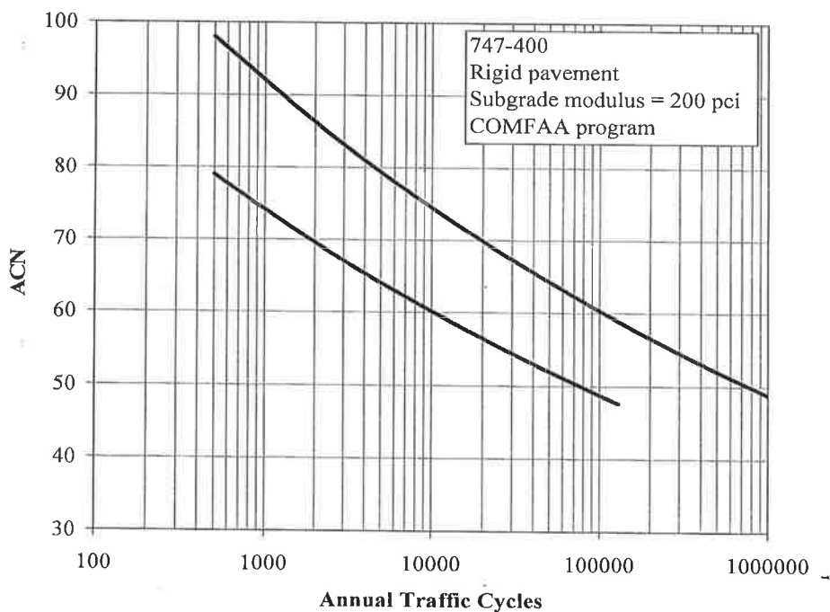
Figura A3-4. Vida Útil con B747-400 en Pavimento Rígido Versus ACN
