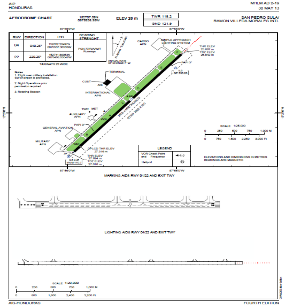
Figura A-1. Ejemplo de un plano de aeródromo que muestra la manera de representar los lugares críticos.
